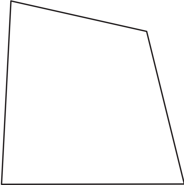
trapezium
