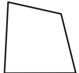
trapezium
